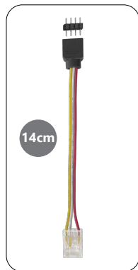
Connettore rapido per controller e strisce LED CCT 927073 CR24CCT
